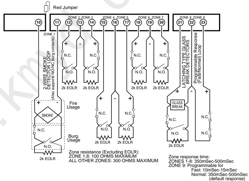
图 8: 防区 1-9 连线图
