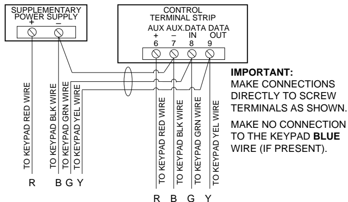
图 7: 键盘另外供电
